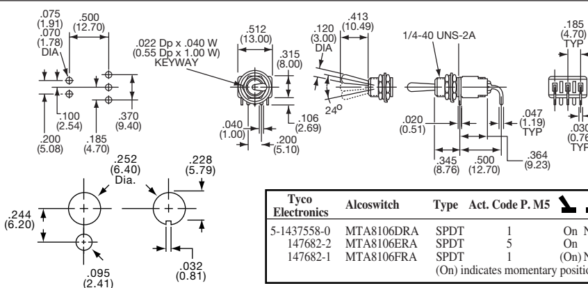
Horizontal Actuation
