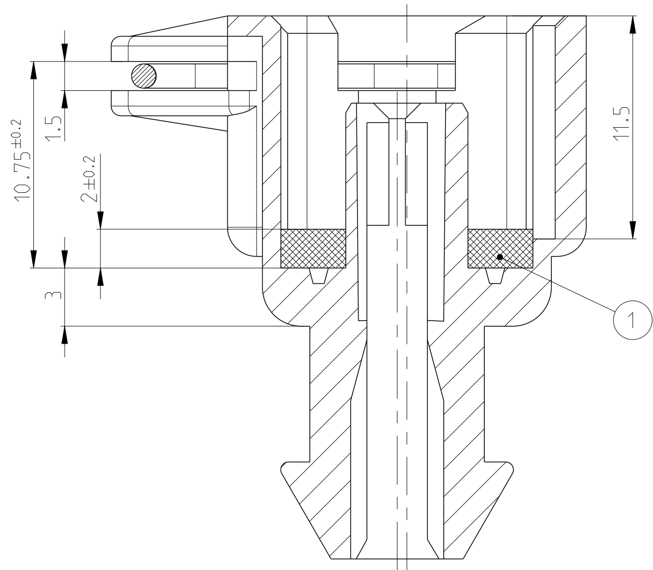
Schnitt SECTION A-A
