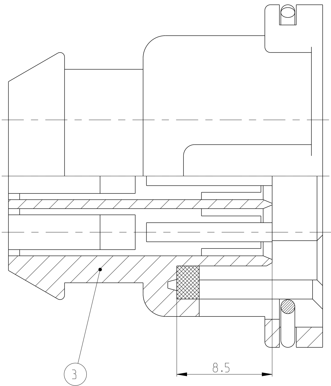
Schnitt SECTION C-C
