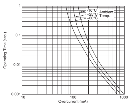
PRG15BC220MM1RC
