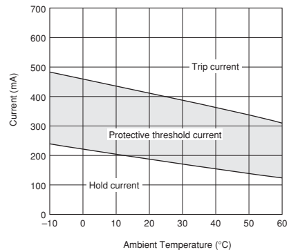
PRG18/21BC3R3M Type
