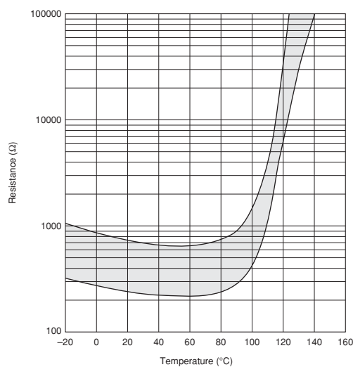
PRF18BB471RB5RB
