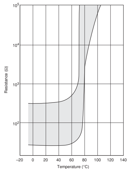
PTF_04BF222Q Type
