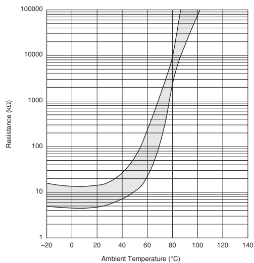
PRF15BG103RB6RC
