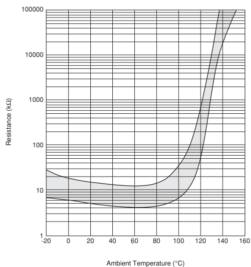
PRF15BB103RB6RC
