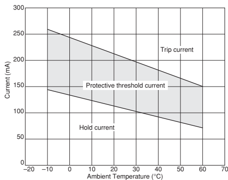
PRG15BC3R3MM1RC
