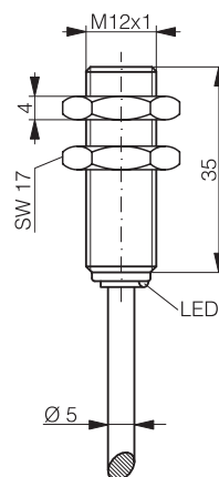
grosser Schaltabstand grosser Schaltabstand
