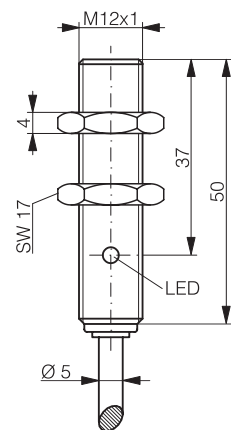
grosser Schaltabstand grosser Schaltabstand
