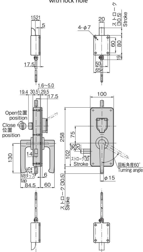
〔A-375-3A-ST 錠前取付け用〕 with lock hole
