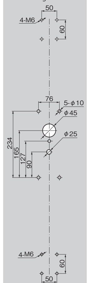
パネル穴明け寸法 Panel drilling dimensions
