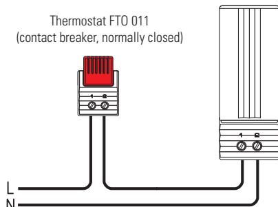
Heater CSK 060
