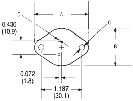
TO-3
