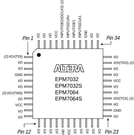
44-Pin TQFP
