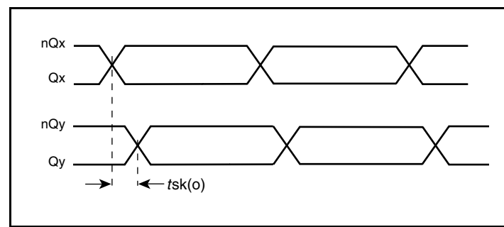
Output Skew
