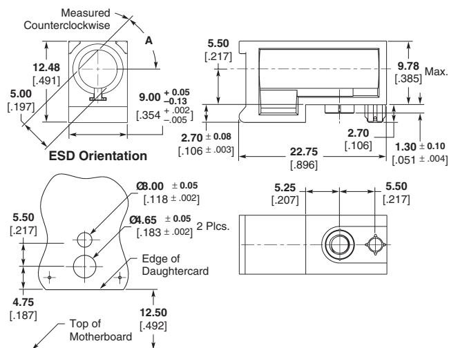
Guide Module Part Number 1469492-X
