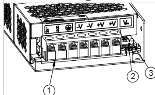
PMC-24V150W1BJ: IP20 Terminal
