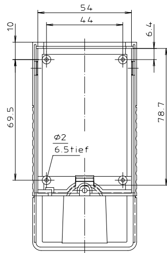
Unterteil von Innen
