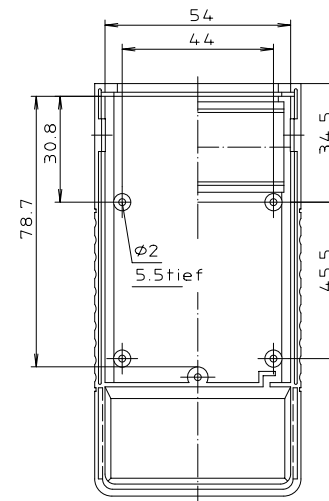
Oberteil von Innen
