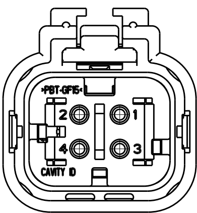
776487-4 SCALE 2:1
