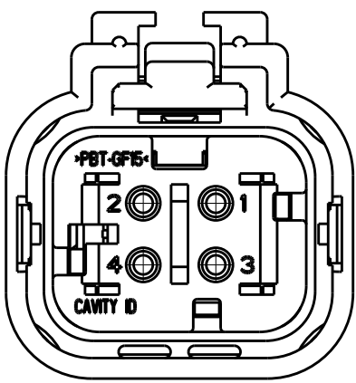
776487-2 SCALE 2:1
