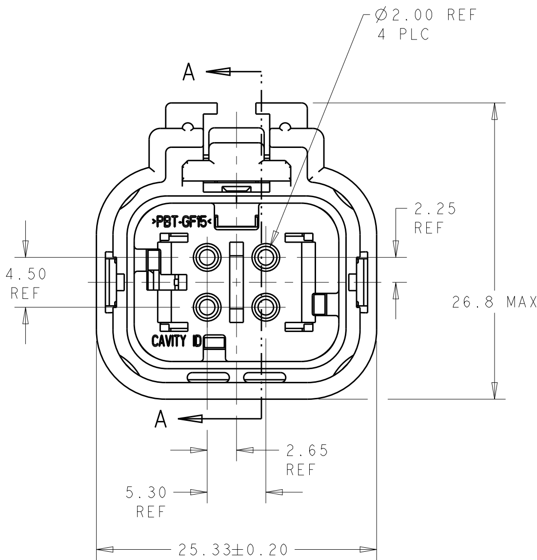
776487-1 SHOWN
