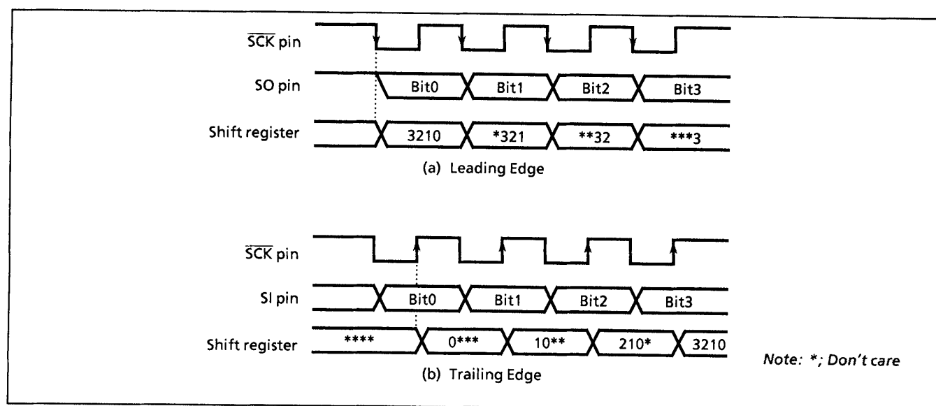
Figure 2-39. Shift Edge
