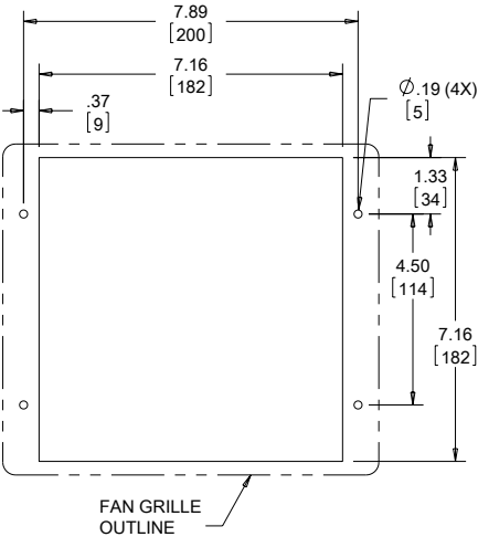
CUTOUT DIMENSIONS
