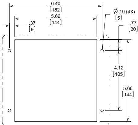
CUTOUT DIMENSIONS
