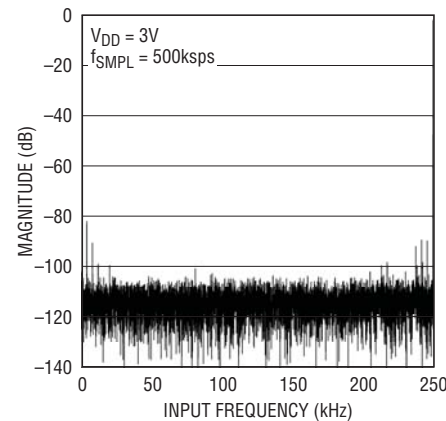
248kHz Sine Wave 8192 FFT Plot
