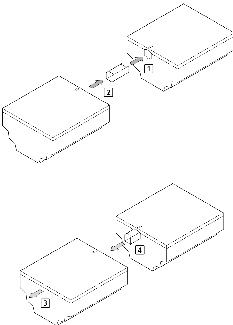
Abbildung 6: Erweiterungen anschließen
