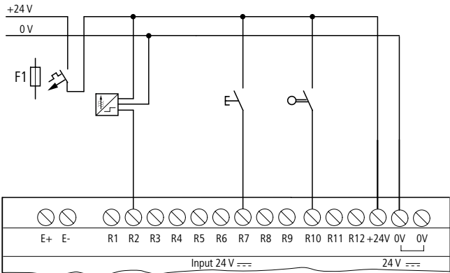
EASY...-DC-.D
