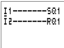
S1 Schließer an I1 S2 Öffner an I2
