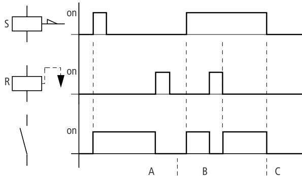
Abbildung 45: Wirkdiagramm verklüpfte Relais
