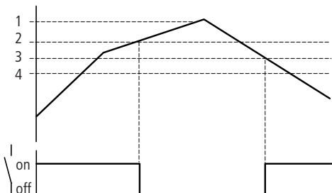
Abbildung 49: Wirkdiagramm Analogwertvergleichler Betriebsart „kleiner als“
