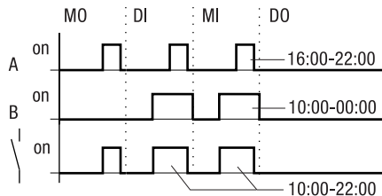
Abbildung 62: Wirkdiagramm „Zeitüberschneidungen“
