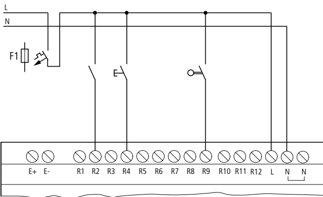
Abbildung 13: Digitale Eingänge anschließen EASY...-AC-E
