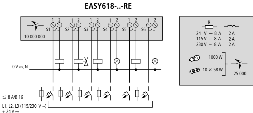
Abbildung 30: Relais-Ausgänge EASY618-...-RE
