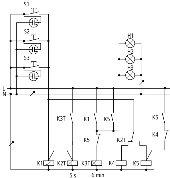
Abbildung 79: Konventionelle Treppenhausbeleuchtung
