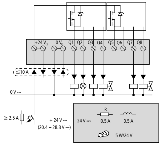
Abbildung 32: Transistor-Ausgänge EASY7...-T..
