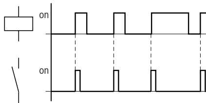
Abbildung 43: Wirkdiagramm Zyklusimpuls bei positiver Flanke
