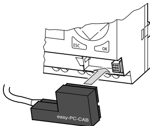
Abbildung 91: EASY-PC-CAB stecken
