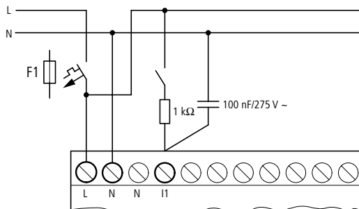
Abbildung 16: Begrenzung des Eingangsstromes durch Widerstand
