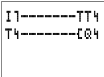
Schaltplandarstellung
