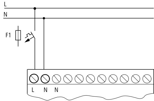
Abbildung 7: Versorgungsspannung an AC-Basisgeräte
