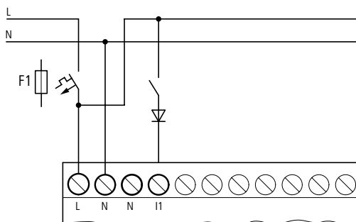
Abbildung 14: AC-Eingang mit Entstörungsschaltung easy-AC und easy-AB
