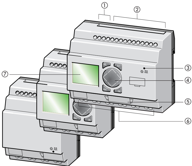
Abbildung 2: Geräteübersicht
