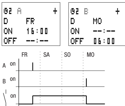
Abbildung 60: Wirkdiagramm „Wochenende“
