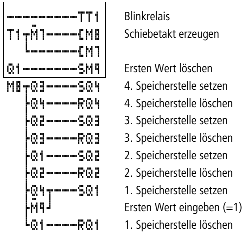
Abbildung 78: easy-Schaltplan Laufflicht
