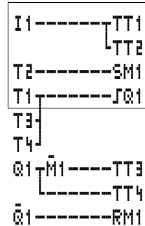
Abbildung 81: easy-Schaltplan Treppenhaus
