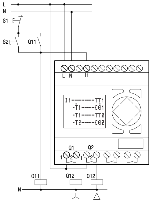
Abbildung 75: Stern-Dreieckschaltung mit easy
