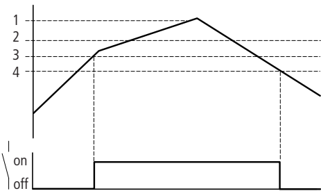
Abbildung 52: Wirkdiagramm Analogwertvergleich der Betriebsart „größer gleich“
