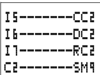
easy-Schaltplan mit Zählerrelais
