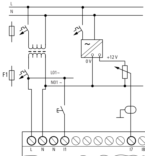
Abbildung 20: easy-AB analoger Eingang, Verbindung der Bezugspotentiale
