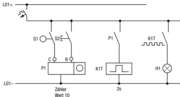
Abbildung 46: Festverdrahtung mit Relais
