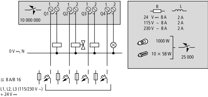
Abbildung 28: Relais-Ausgänge EASY512-...-R..
