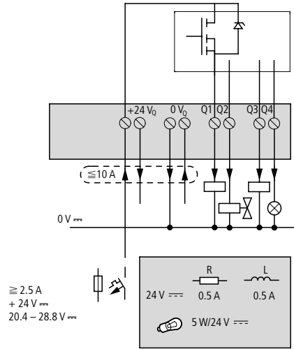
Abbildung 31: Transistor-Ausgänge EASY512-...-T..
