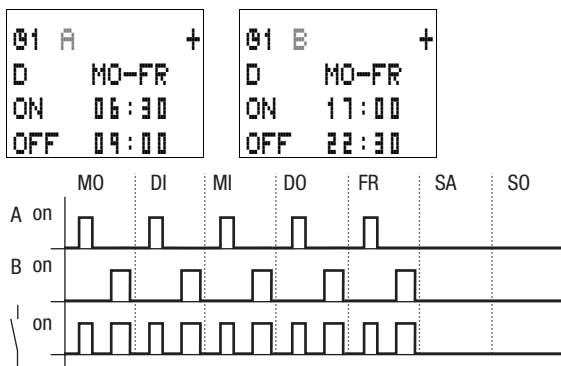
Abbildung 59: Wirkdiagramm „Arbeitstage“
