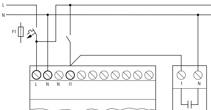
Abbildung 17: easy mit EASY256-HCI
