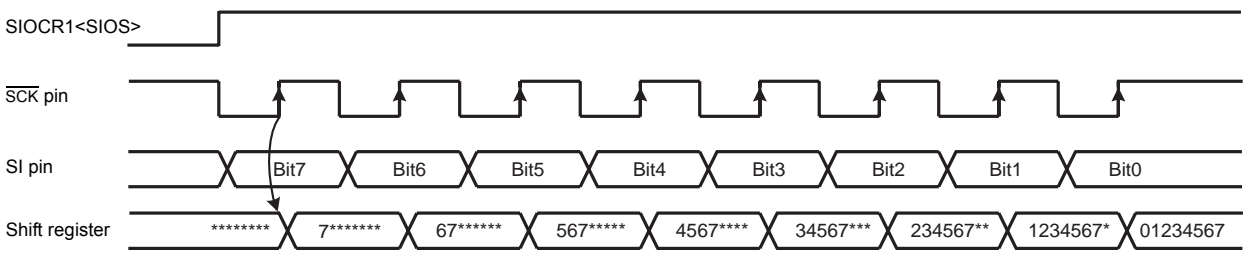
Figure 11-4 Shift Edge
