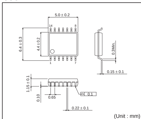
SSOP-B14
