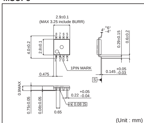
MSOP8
