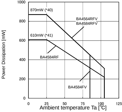
(d)BA4564R/BA4584/BA4584R family
