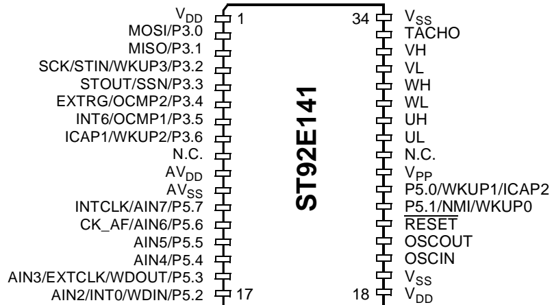
SO34 Package
