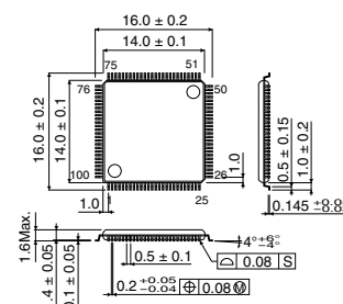
VQFP100
