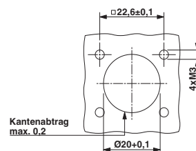
Einbaumaße: RF-1.S..8AAC00, RF-1.P..8AAC00
