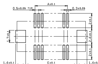
基板取付け寸法 MOUNTING LAYOUT
