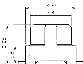
吸着テープ位置 POSITION OF VACUUM TAPE
