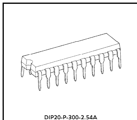
DIP20-P-300-2.54A
