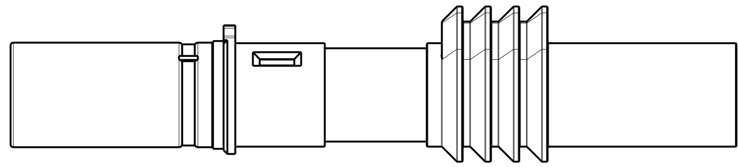
1445693-3, -4 & -5 SCALE 4:1
