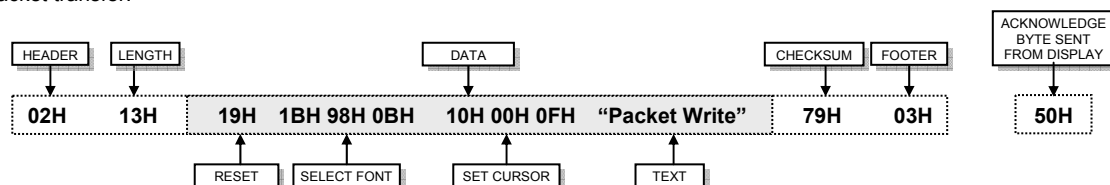
Packet format.
