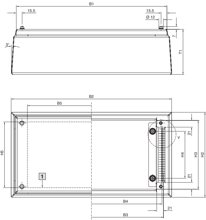
1 Max. Einbaufäche Deckel
