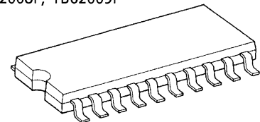
SOP20-P-300-1.27
