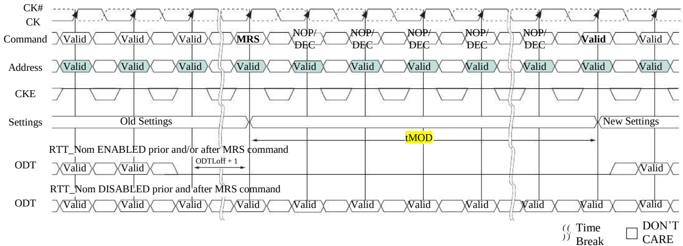
Figure 2.3.1b tMOD Timing
