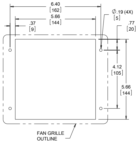
CUTOUT DIMENSIONS
