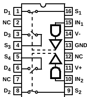
HI-390 (CERDIP) TOP VIEW
