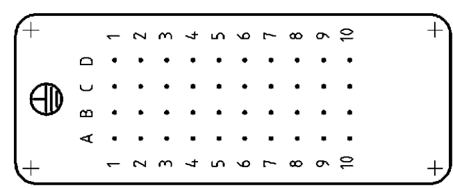
Kontaktanordnung Contact arrangement Ansicht Anschlußseite view from termination side
