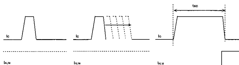
Fig.3 短絡保護遅れ時間 ( t_{SC} ) の定義
