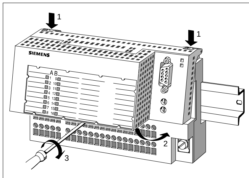
Bild 2-3 Elektronikblock montieren
