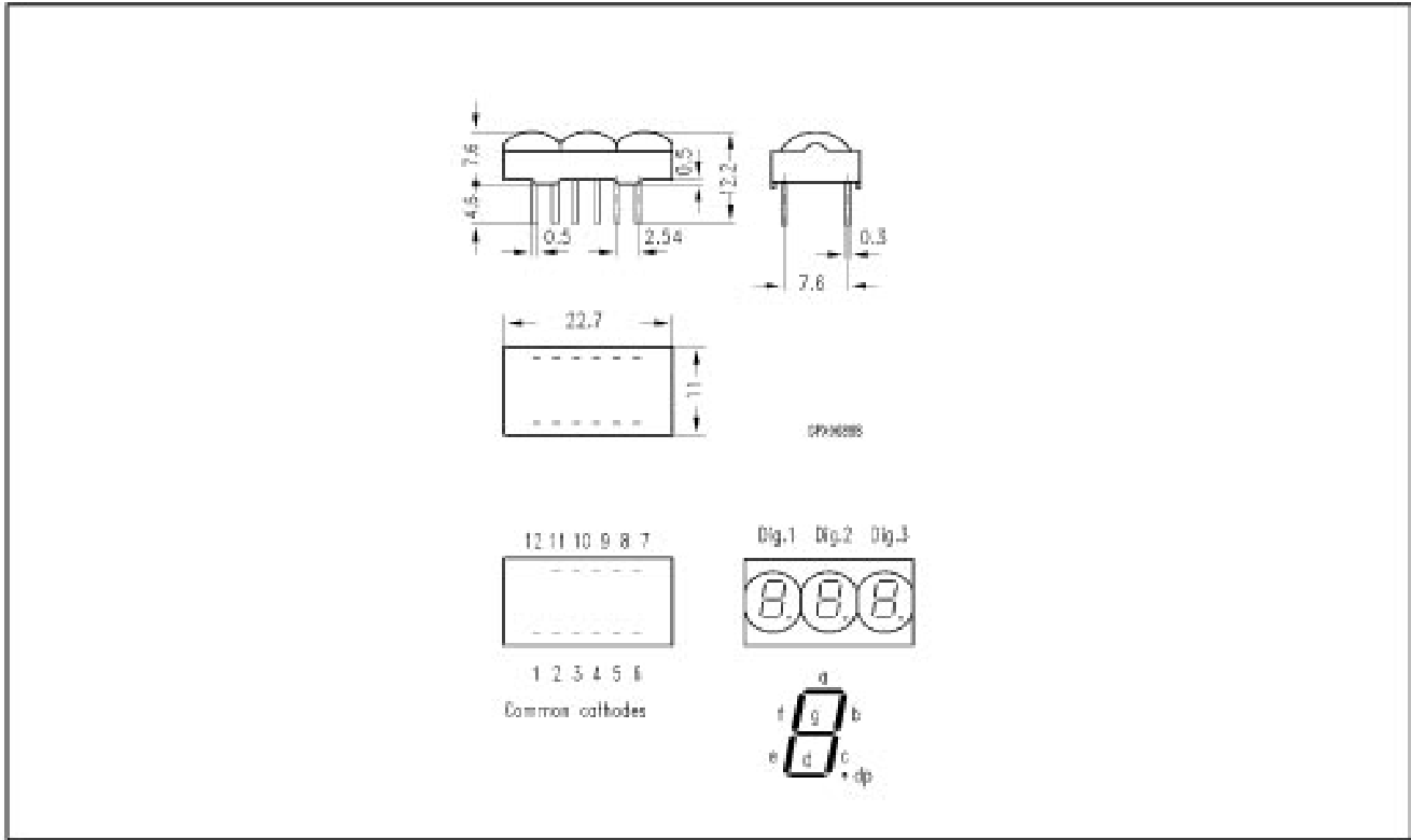
DL-430 M
