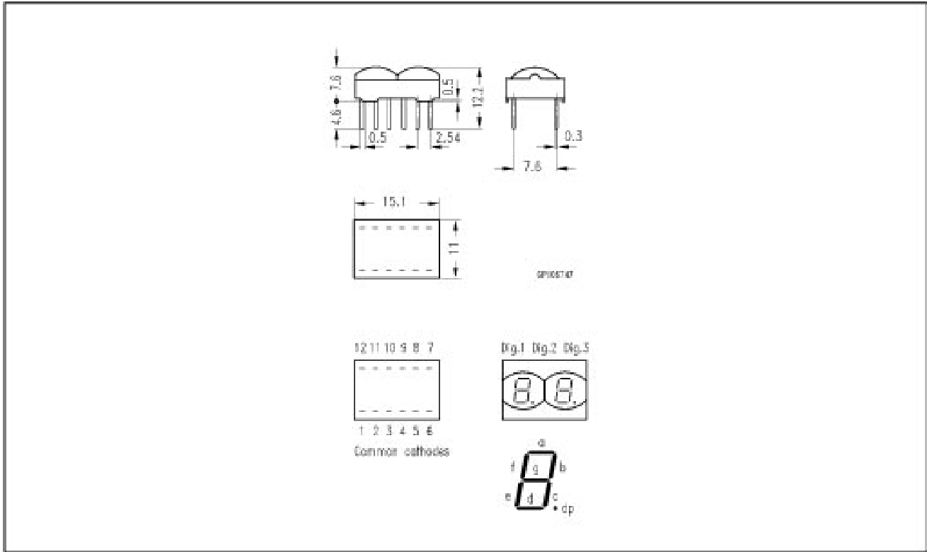
DL-440 M
