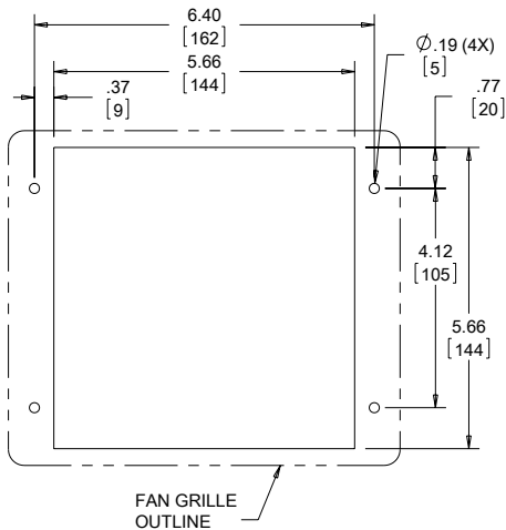
CUTOUT DIMENSIONS
