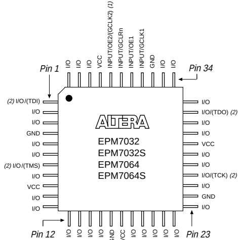
44-Pin TQFP
