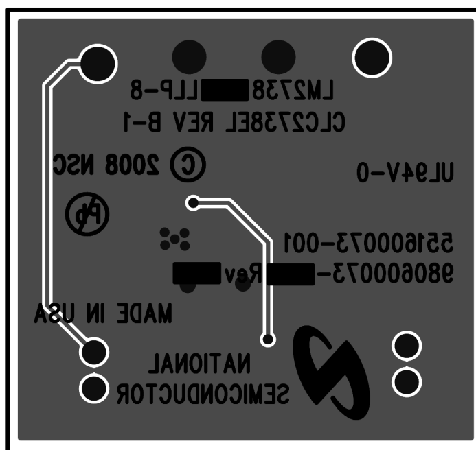
Figure 3-4. Bottom Layer
