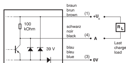
NPN
