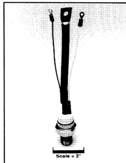
T600 Phase Control SCR 150-175 Amperes, 100-1600 Volts
