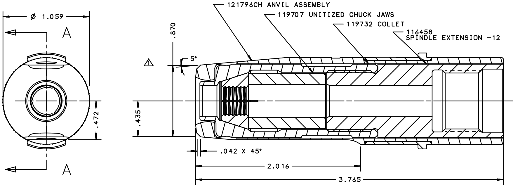
SECTION A-A
