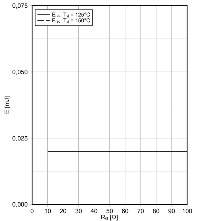
Schaltverluste Diode, Brems-Chopper (typisch) switching losses Diode, Brake-Chopper (typical) E_{rec} = f(R_G) I_F = 40\ \text{A} , V_{CE} = 300\ \text{V}
