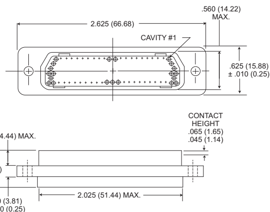
Receptacle
