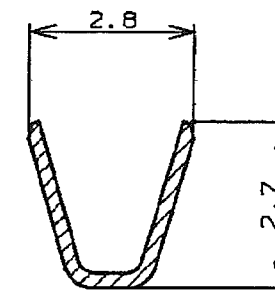
断面 "D"- "D" (SECT)
