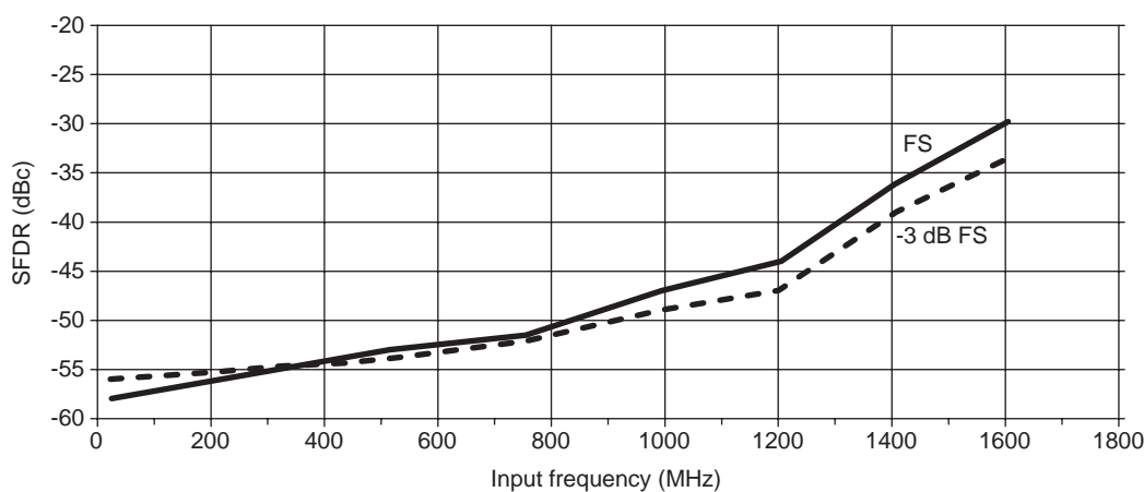
Figure 18. SFDR (dBc)
