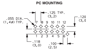
PN41LGSA02QE 4PDT
