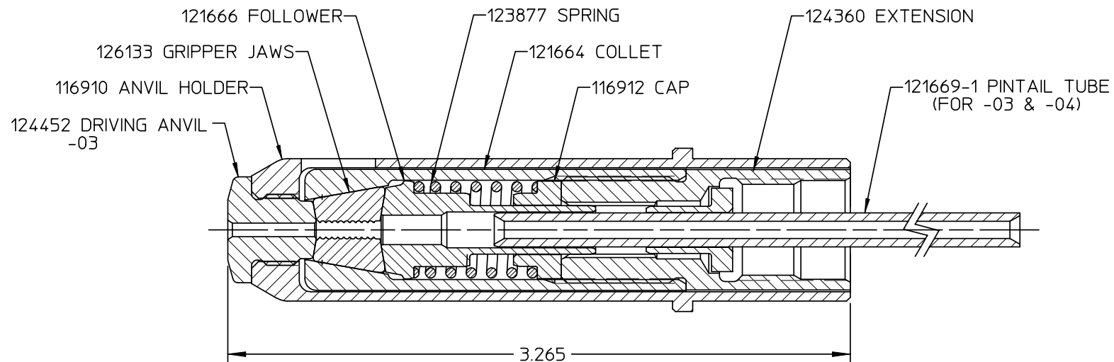
SECTION A-A
