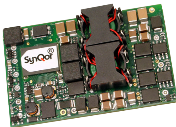
IQ65033QMA10 Module
