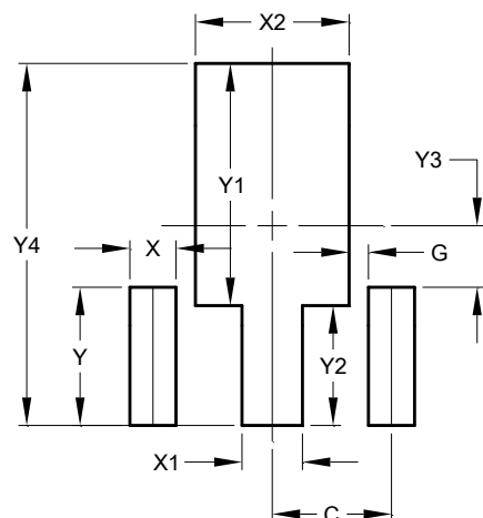
SOT89
