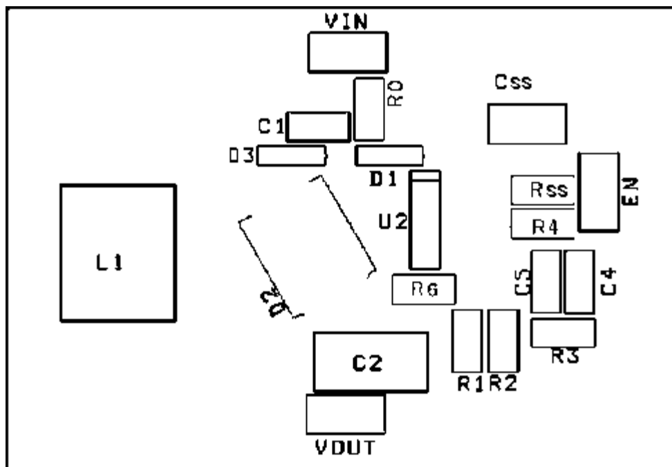
(Componet Side - TOP)
